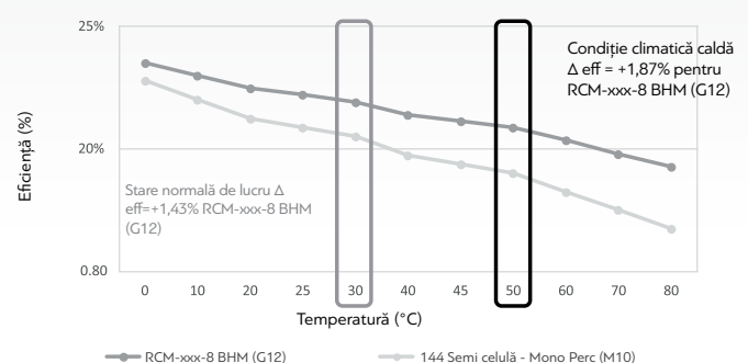
Evoluția eficienței energetice, la temperaturi ridicate
