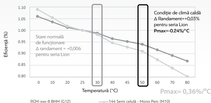
Evoluția randamentului, la temperaturi ridicate
